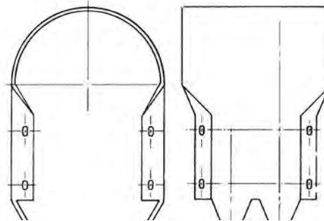
RETURN CAP TYPE TA
